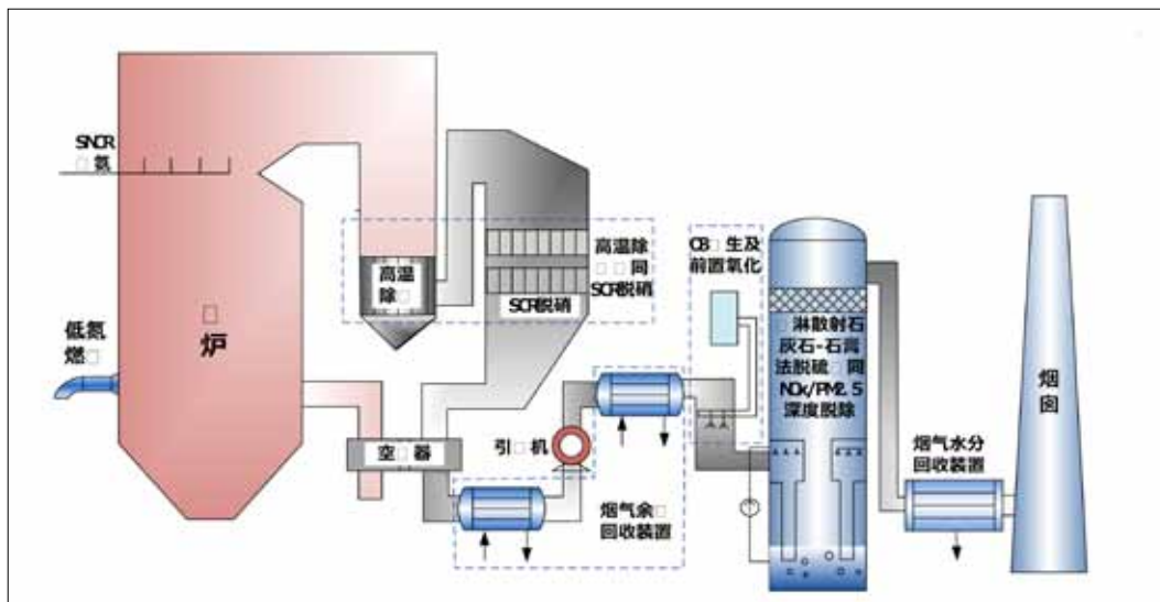
高温除尘器工作原理
